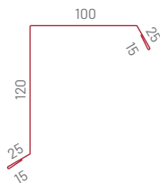
Závětrná lišta boční F02
