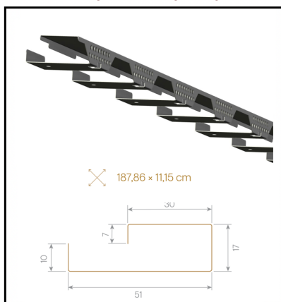
F68- Větrací pás hřebene pro trapéz T14
