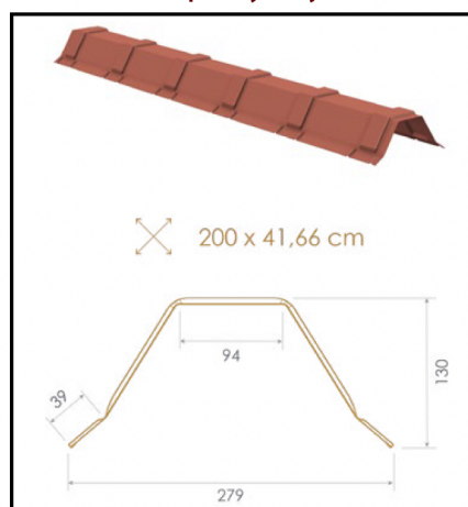
F73 - Hřebenáč trapezový velký s embosováním
