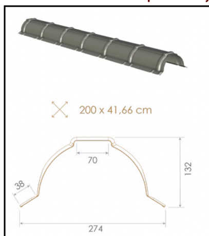
F72 - Hřebenáč k taškovému profilu velký
