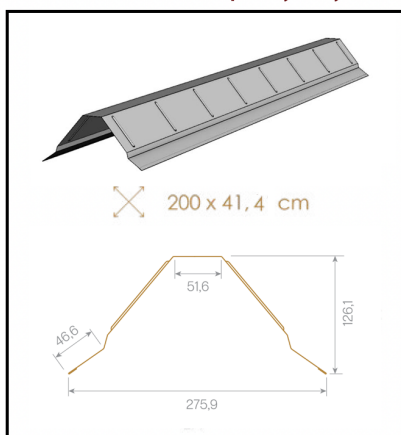
F82 - Hřebenáč trapezový velký
