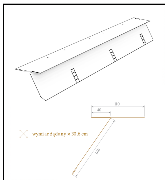
F84- Nadokapový pás SnapLock Quattro
