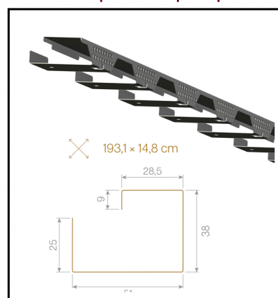
F70- Větrací pás hřebene pro trapéz T35
