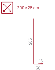
Podokapní tvarovka čelní desky F10
