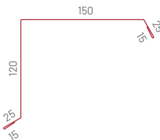
Závětrná lišta boční F02
