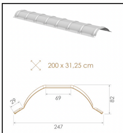
F71 - Hřebenáč k taškovému profilu malý
