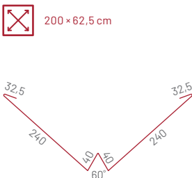
Úžlabí s můstkem F12
