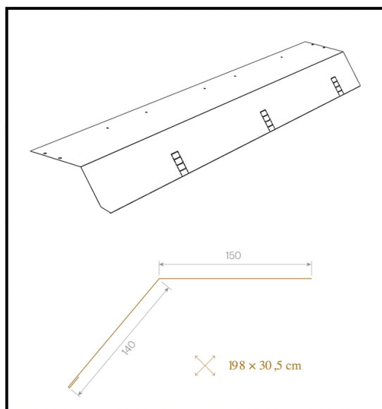
F83- Nadokapový pás Quattro
