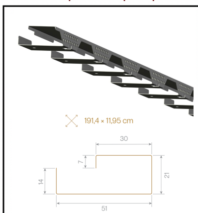
F69- Větrací pás hřebene pro trapéz T18
